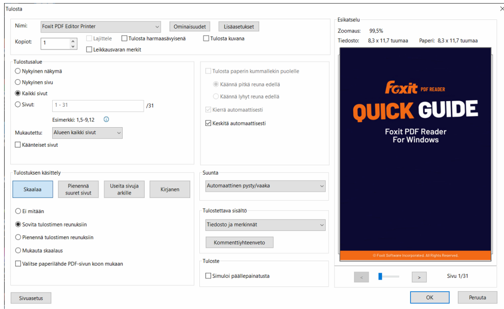
Tulosta-valintaikkuna
