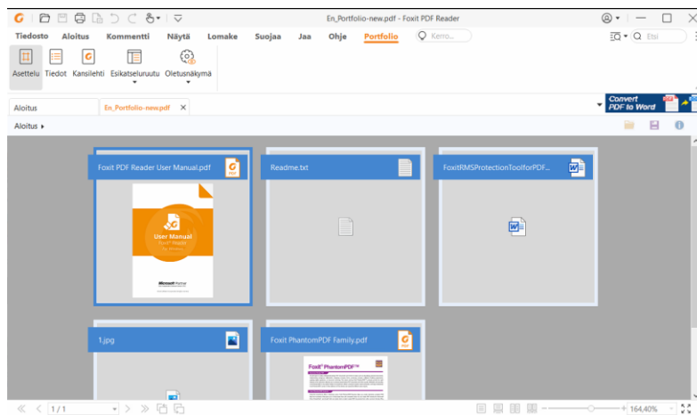
Esimerkki PDF-portfoliosta
