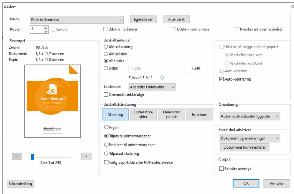
Dialogboksen Udskriv
