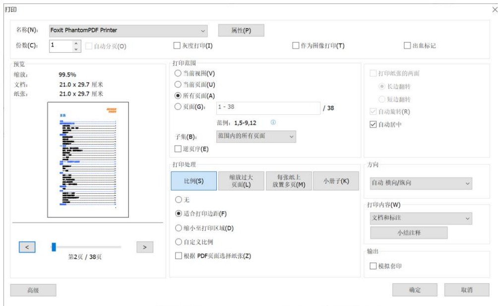
打印对话框
