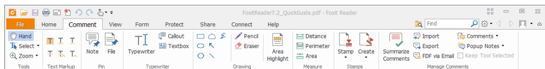
Fig. 4 Comment Tab
