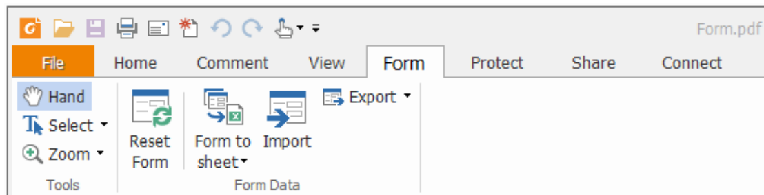
Fig. 6 Form Tab
