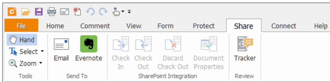
Fig. 8 Share Tab
