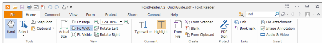
Fig. 3 Home Tab
