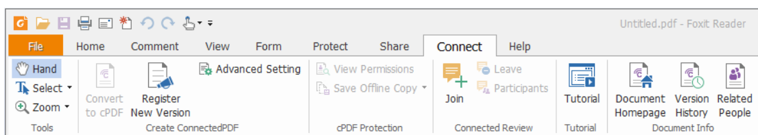
Fig. 9 Connect Tab
